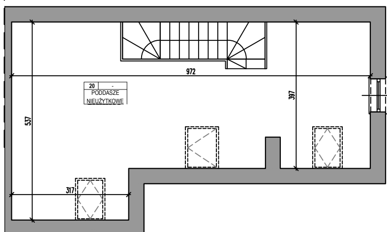
RZUT PODDASZA
