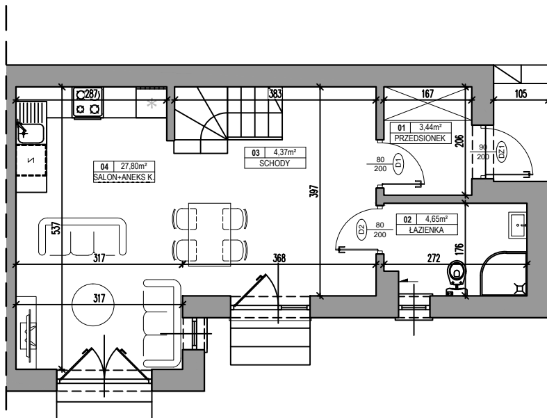
RZUT PARTERU
