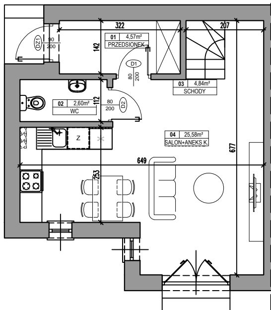
RZUT PARTERU
