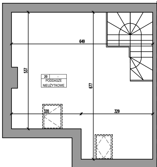
RZUT PODDASZA
